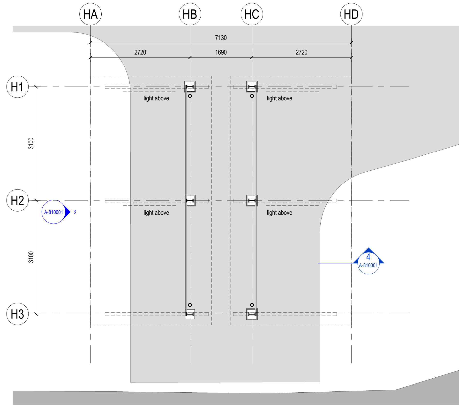
2 Hat Stand Floor Plan 1 : 50
