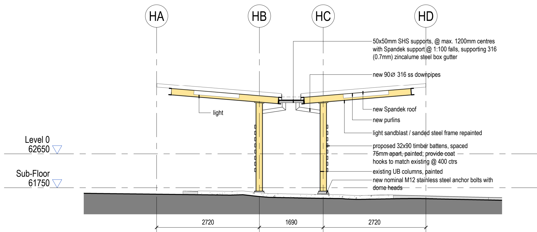
4 Hat Stand Section 1 : 50
