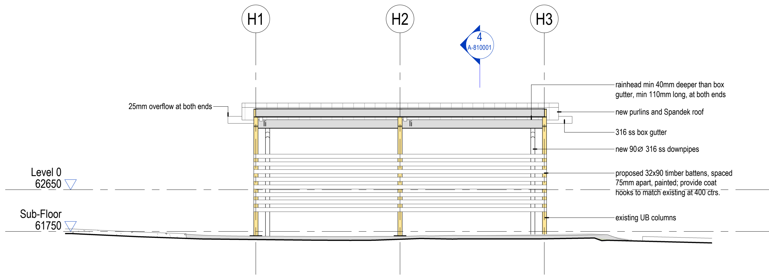
3 80 N Hat Stand Elevation 1 : 50
