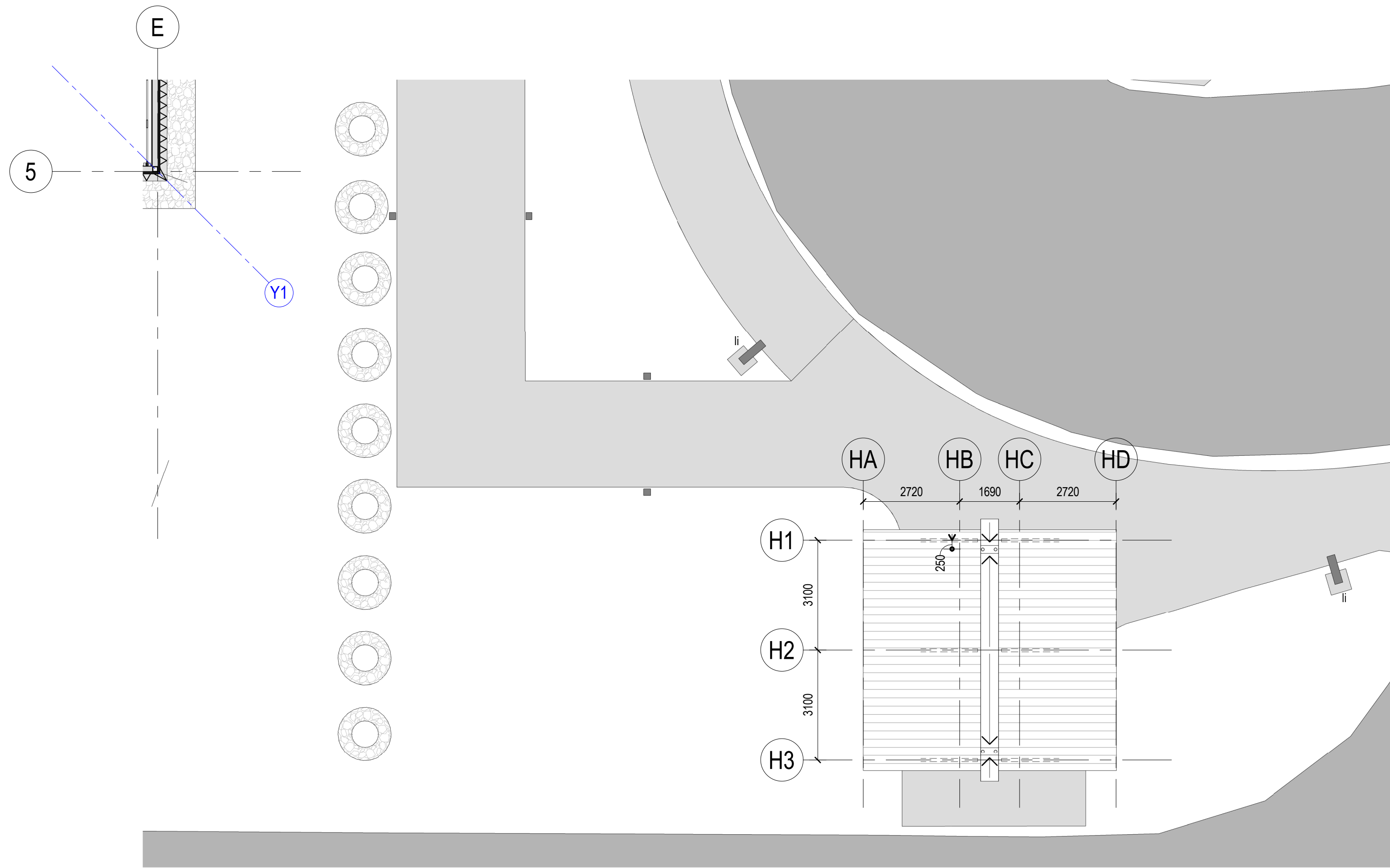
1 Hat Stand Site Plan 1 : 100
